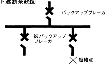
カスケード遮断系統図
