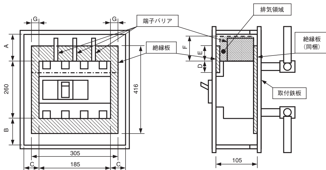
裏面形
