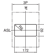
パネル切抜寸法図 (正面図)
