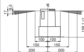
パネルヒンジ位置 (斜線部) (底面図)
