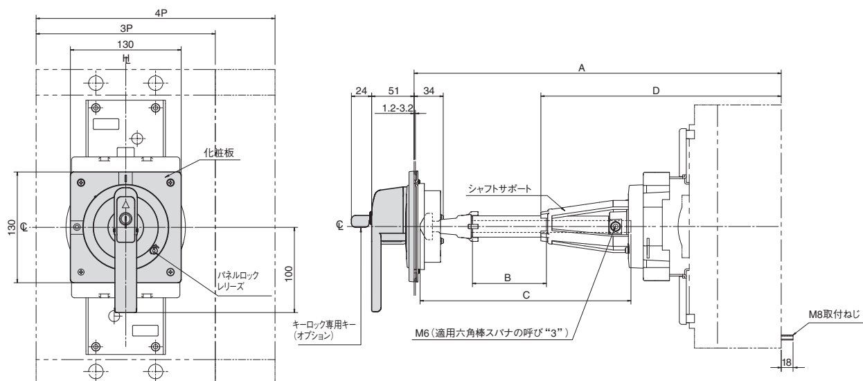
●外形寸法図
