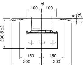
パネルヒンジ位置（斜線部） （底面図）
