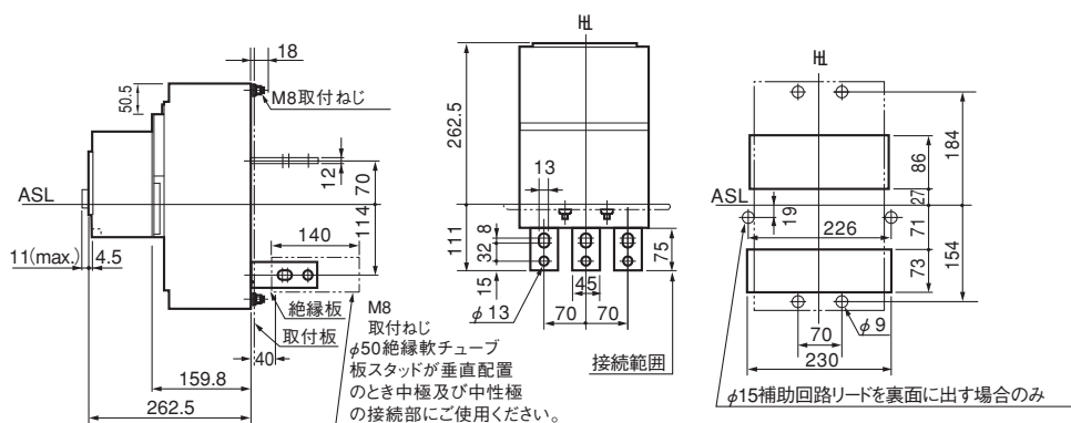
(下面図)
