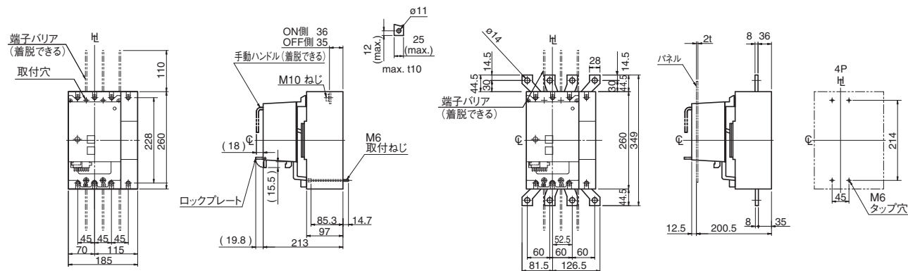
端子バー付 (オプション)
