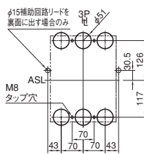
取付寸法図 (正面図)
