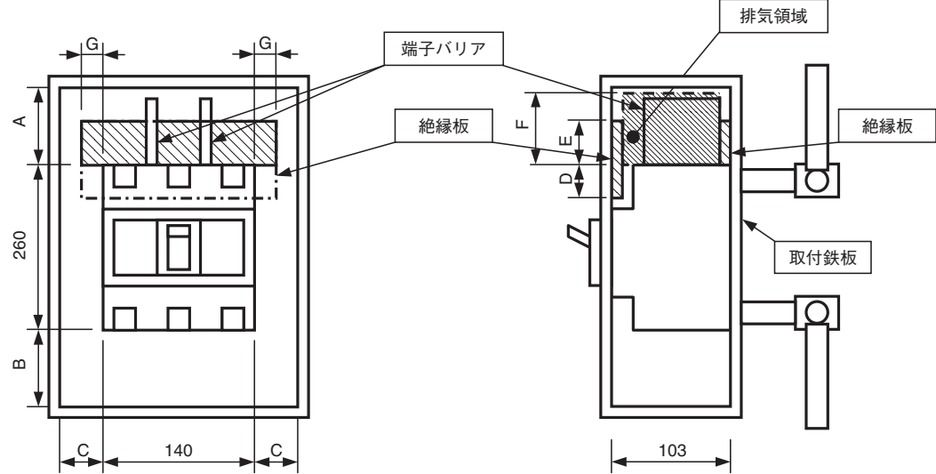
裏面形
