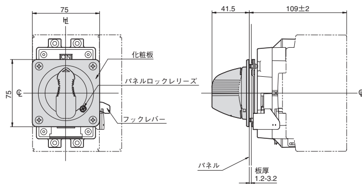
●外形寸法図
