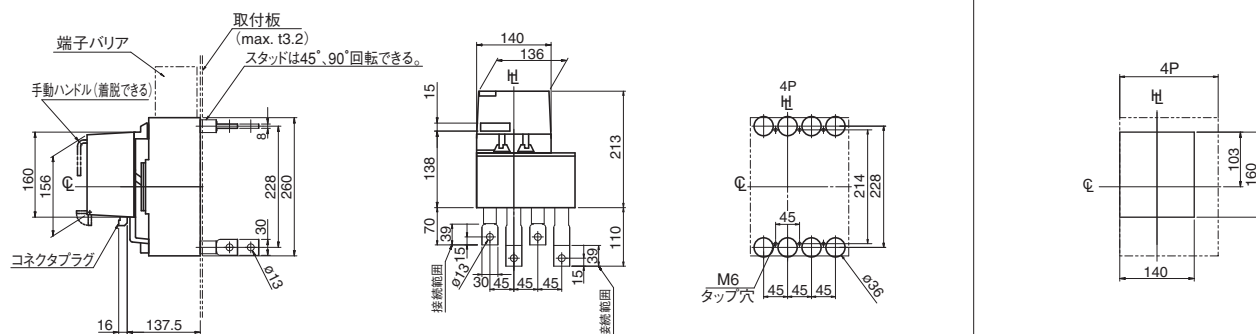
(下面図)
