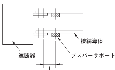
水平端子の場合
