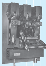
【AA-10形1000A 3P固定形】
