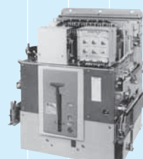
【AP-20形2000A 3P引出形】
