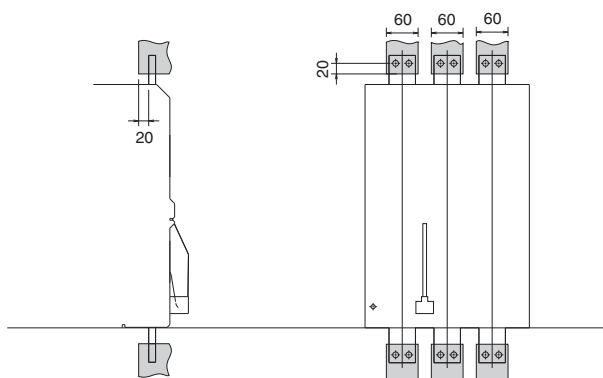
右側面図
