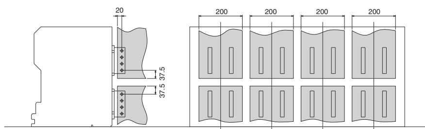
右側面図
