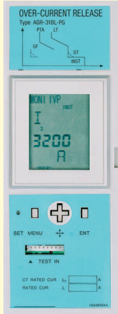
LCD表示式高機能OCR AGR-31B形
