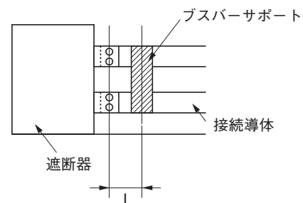
垂直端子の場合
