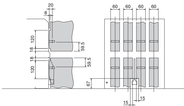
右側面図
