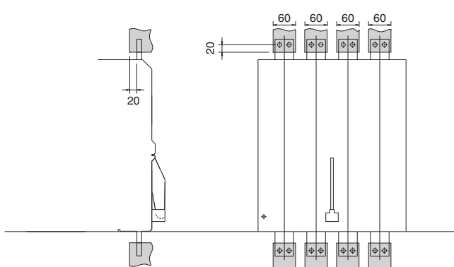
右側面図
