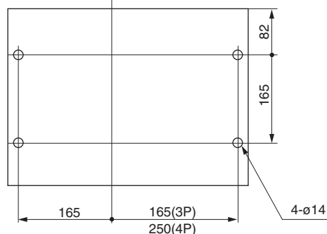
取付穴
