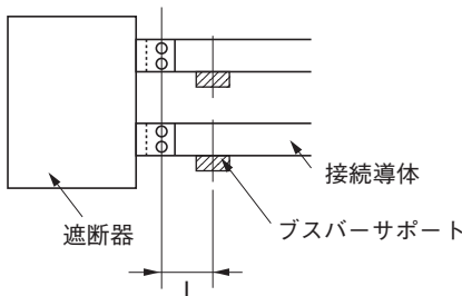
垂直端子の場合
