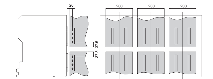
右側面図
