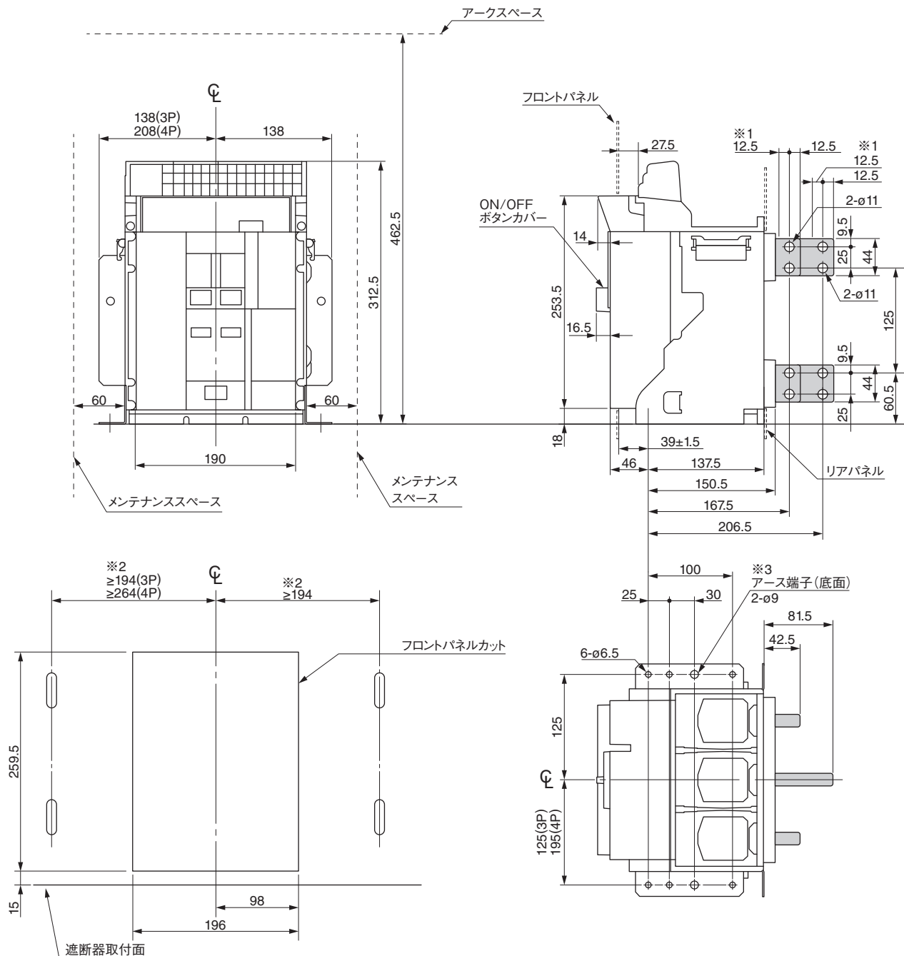
パネル切抜寸法図(表面)
