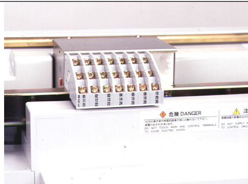
図5 制御回路端子
