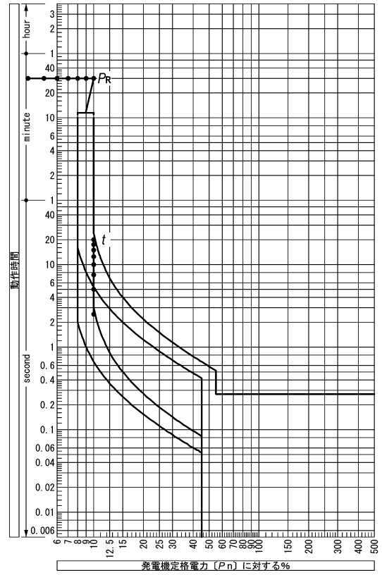
図31 AGR-31BS (S特性) 形OCRの特性
