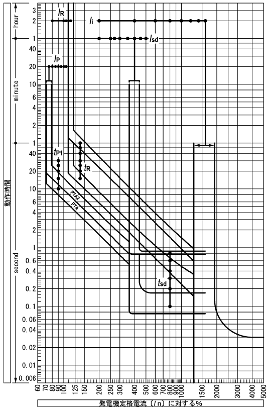
図31 AGR-31BS (S特性) 形OCRの特性
