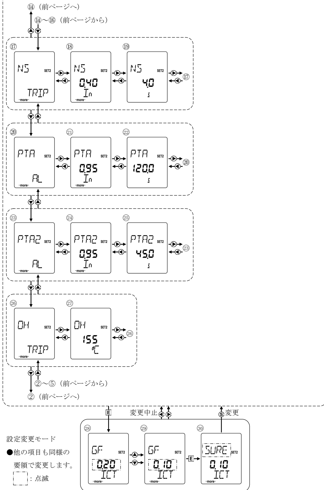
図 4 0 - 2 特性値の表示・変更要領 2
